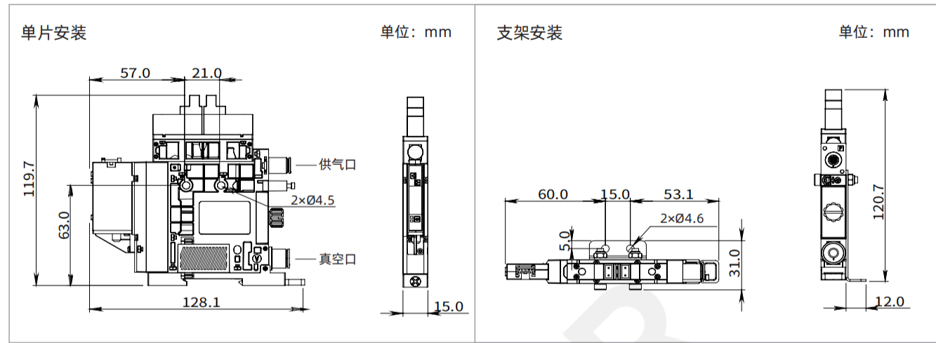
外形尺寸图
