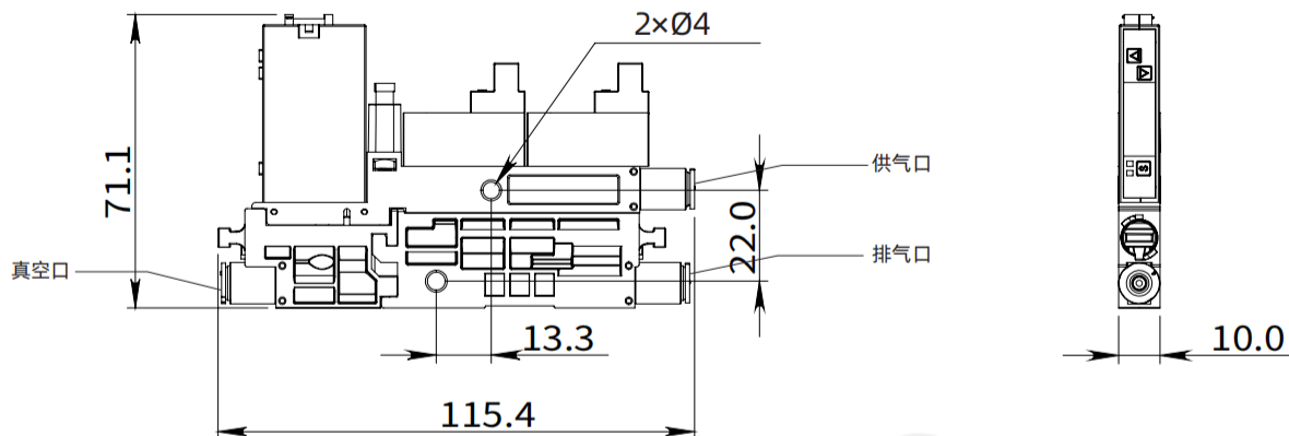
外型尺寸图
