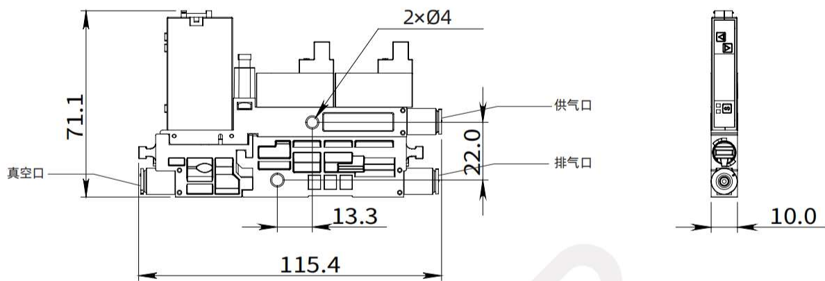
外型尺寸图
