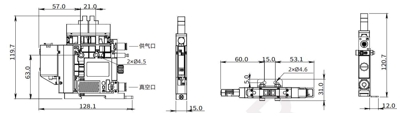
单片安装
