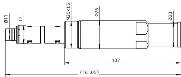
VHD17-HB-3 尺寸图
